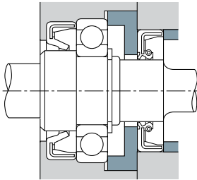
Fig. 11.8 Exemplo de Retentores (1)
