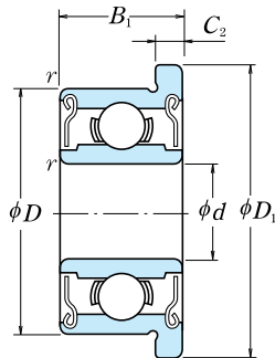
Blindado ZZ - ZZS
