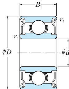
Blindado ZZ - ZZ1
