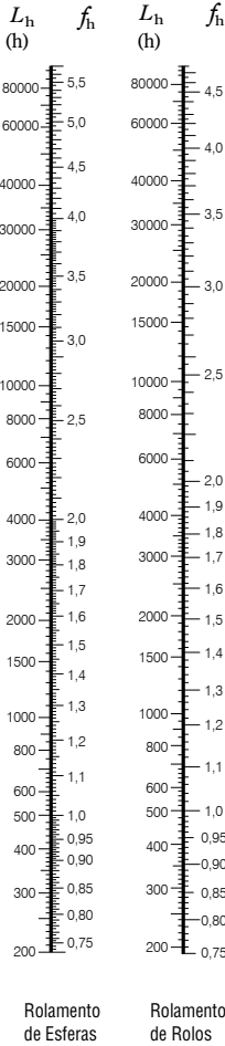
Fig. 5.4 Vida Nominal e Coeficiente de Vida
