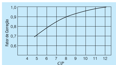
Fig. 6.1 Correção do Limite de Rotação devido à Intensidade da Carga no Rolamento
