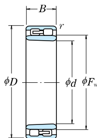
Tipo NNU Furo Cônico
